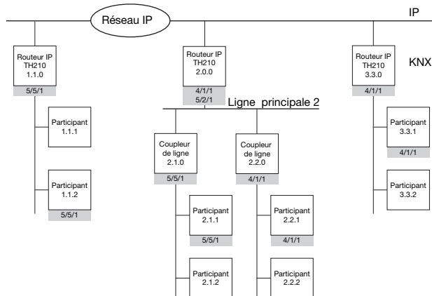
Illustration 1 : Routeur IP/KNX TH210 utilisé en coupleur de zones et coupleur de lignes
