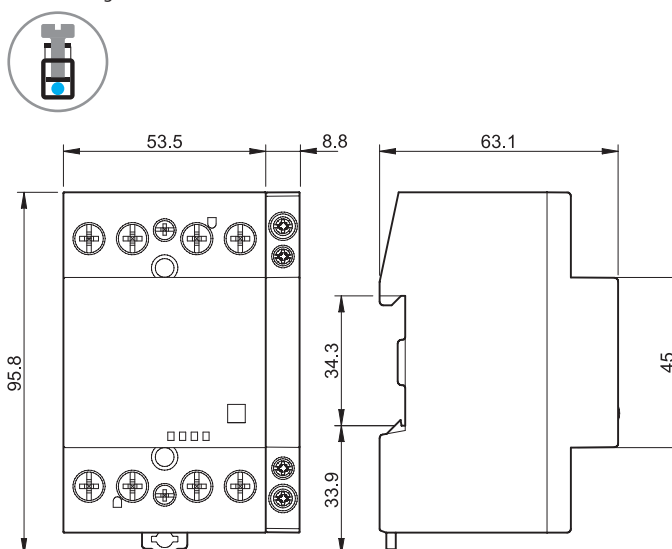
Types 22.44/22.64 + 022.63/022.65 Bornes à cage
