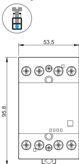
Types 22.44/22.64 Bornes à cage
