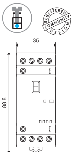
Type 22.34 Bornes à cage
