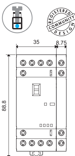
Type 22.34 + 022.33/022.35 Bornes à cage
