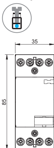
Types 22.74 Bornes à cage
