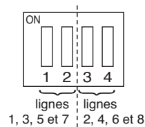
Sélecteurs S1/S2/S3/S4 (un par ligne DAS, ex pour la ligne 5 : 1 et 2 de S1)
