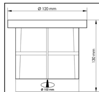
Obturbateur prévu pour le 2 ème presse-étoupe
