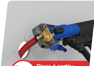
Pince à sertir : profils de sertissage H et RF
