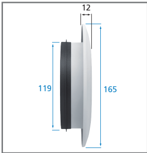
ONDÉA 125
