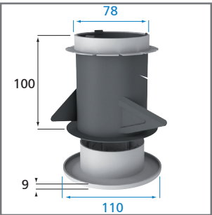
ONDÉA 80 P
