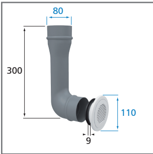
ONDÉA 80 L
