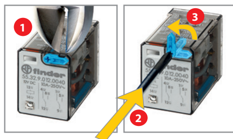
Bouton test verrouillable et indicateur mécanique (0010, 0040, 0050, 0054, 0070, 0074, 0090, 0094)
