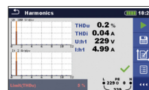
Harmoniques
