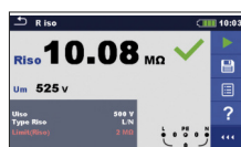
Mesure d'isolement
