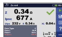
Mesure de terre sans piquet
