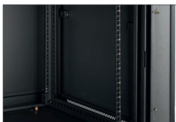
Les montants 19" avant et arrière sont librement ajustables pour faciliter l'installation des équipements.
