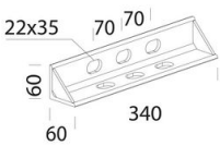
345 Étrier mural
