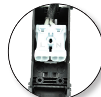
Bornier de raccordement à connexion auto avec repiquage – prêt à poser
