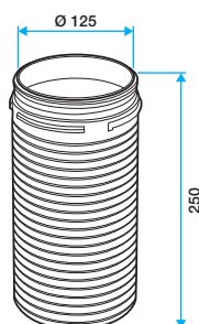
Rallonge circulaire Ø125 mm
