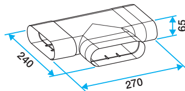
Té 90° horizontal
