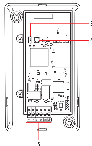
Vue postérieure
