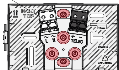
Entrées de câbles
