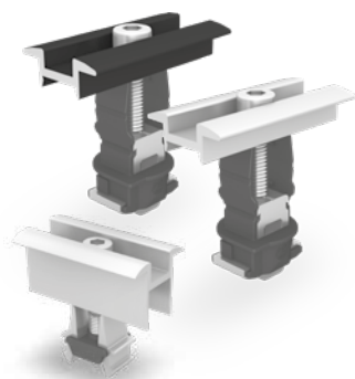
K2 Clamp MC argent/noir Hauteur du cadre du module: 25 - 40 mm
