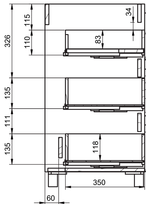
B-B ( 1 : 8 )
