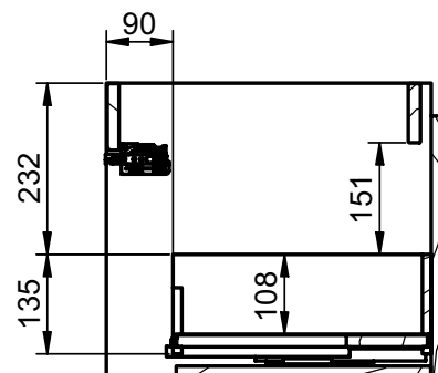
B-B ( 1 : 10 )
