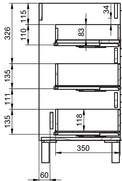
B-B ( 1 : 10 )
