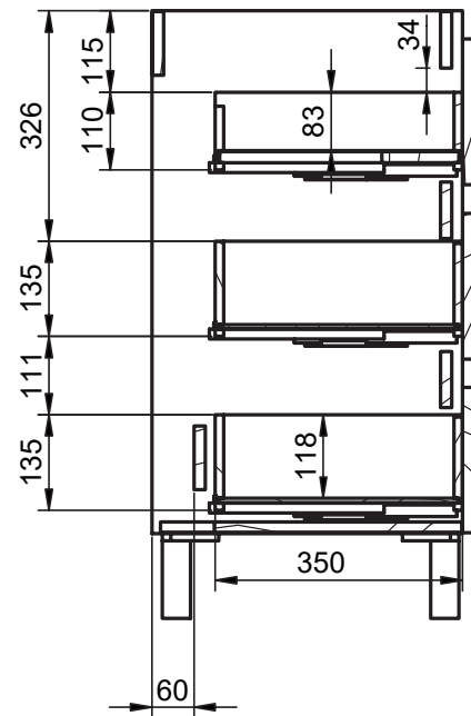
B-B ( 1 : 10 )
