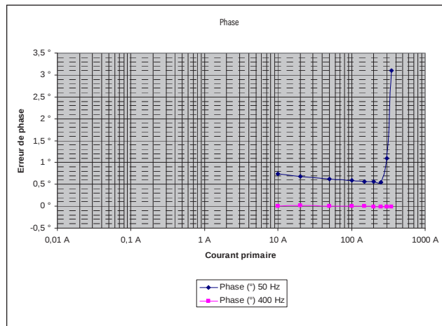
Déphasage typique
