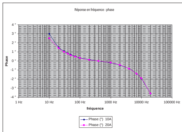
Déphasage typique
