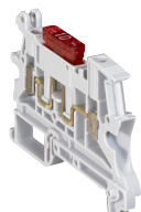
Bloc réf. 0 371 80 avec fusible automobile à languette
