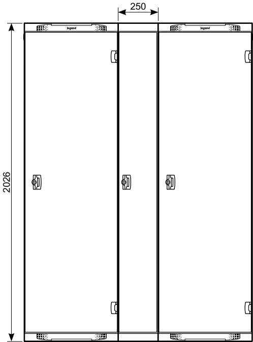
VUE AVANT
