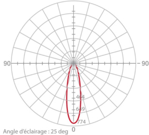
Courbe de distribution de la lumière (unité : cd)
